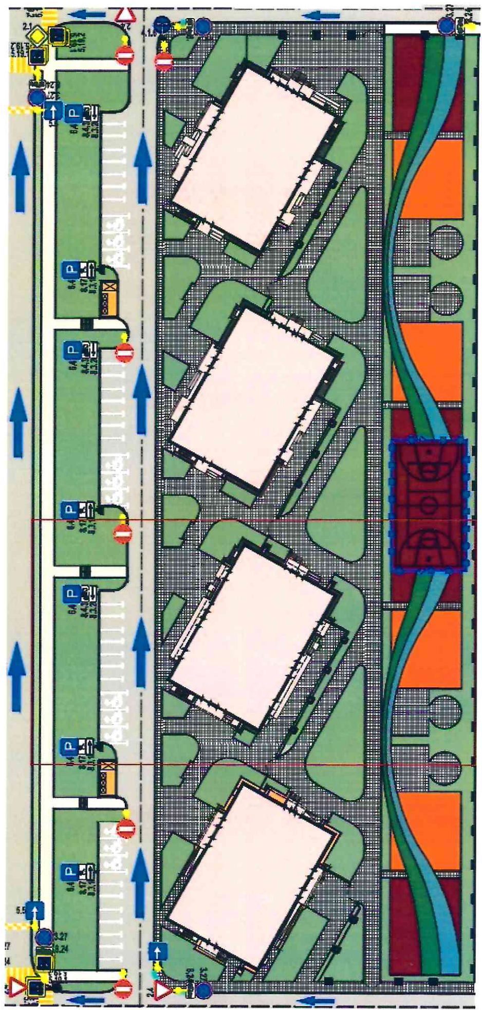
Схема дорожного движения, дорожной разметки и дорожных знаков на придомовой территории
