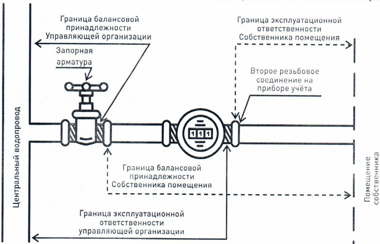
Схема №1. Граница балансовой принадлежности и эксплуатационной ответственности УО при лучевой разводке холодного (в том числе предназначенного для доочистки воды), горячего водоснабжения, в коллекторном узле.
