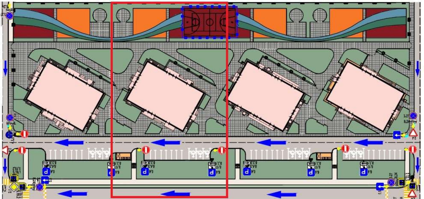
Схема дорожного движения, дорожной разметки и дорожных знаков на придомовой территории
