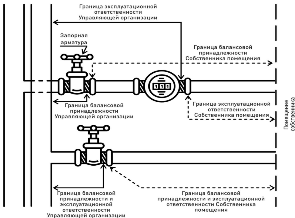
Схема №2. Граница балансовой принадлежности и эксплуатационной ответственности УО при лучевой разводке системы отопления в коллекторном узле.
