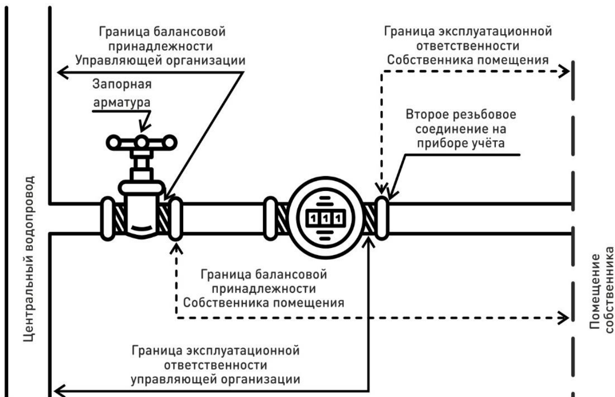
Схема №1. Граница балансовой принадлежности и эксплуатационной ответственности УО при лучевой разводке холодного водоснабжения.
