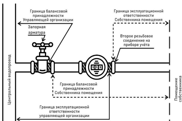
Схема №1. Граница балансовой принадлежности и эксплуатационной ответственности УО при лучевой разводке холодного (в том числе предназначенного для доочистки воды), горячего водоснабжения в коллекторном узле.
